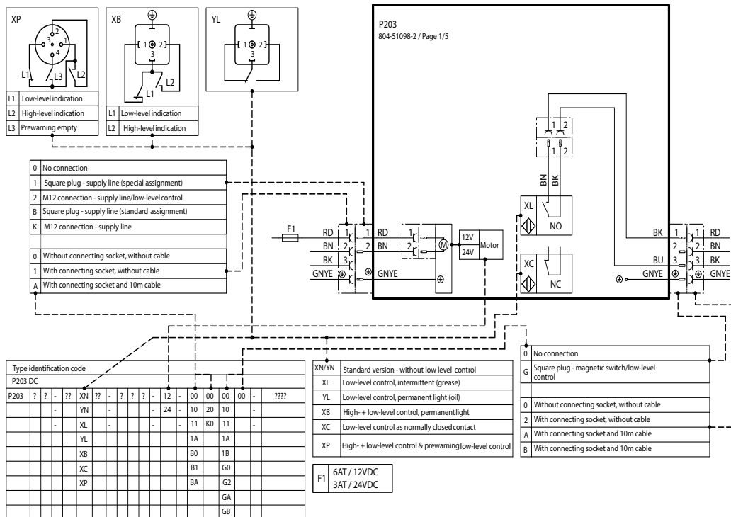
Esquema de conexiones P203 V DC sin pletina de mando Fig. 31
