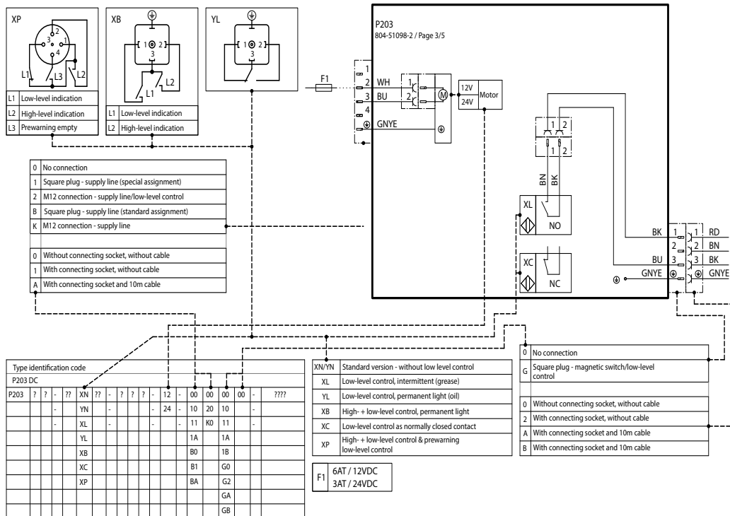
Esquema de conexiones P203 V DC sin pletina de mando Fig. 33
