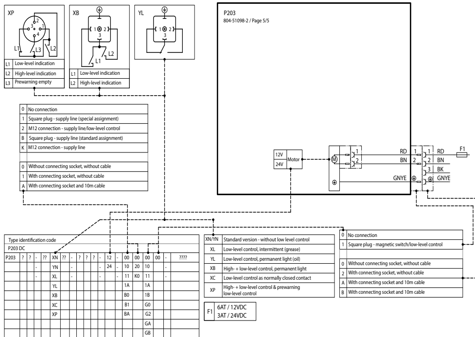
Esquema de conexiones P203 V DC sin pletina de mando Fig. 35
