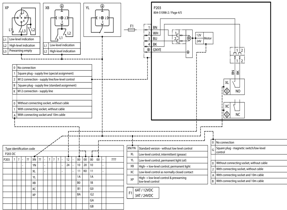
Esquema de conexiones P203 V DC sin pletina de mando Fig. 34
