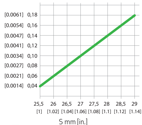
Ajuste del caudal en el elemento de bomba R Fig. 10
