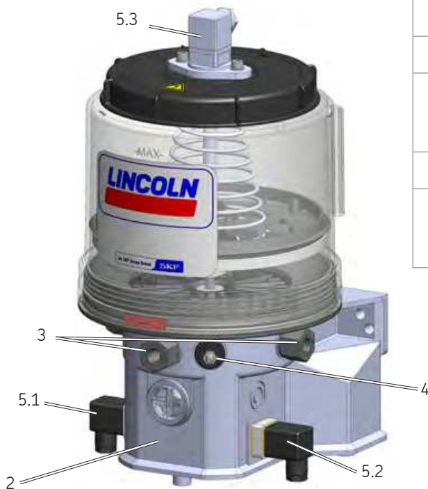
Resumen, descripción de la función de bombas con placa seguidora Fig. 4
