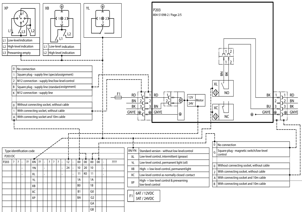
Esquema de conexiones P203 V DC sin pletina de mando Fig. 32
